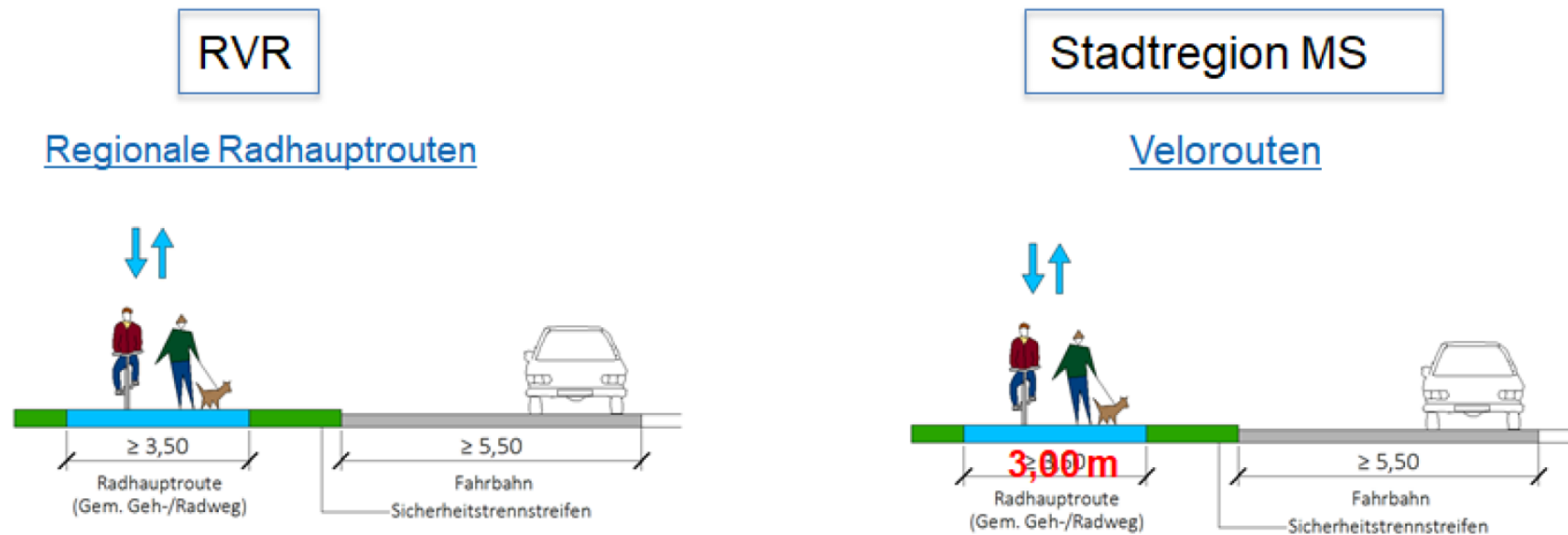
Abb. 3: Musterquerschnitt für die gemeinsame Führung an Hauptverkehrsstraßen außerorts als Radhauptverbindungen
