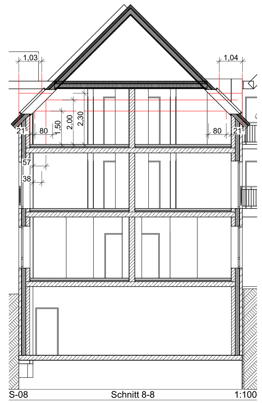
S-08 Schnitt 8-8 1:100
