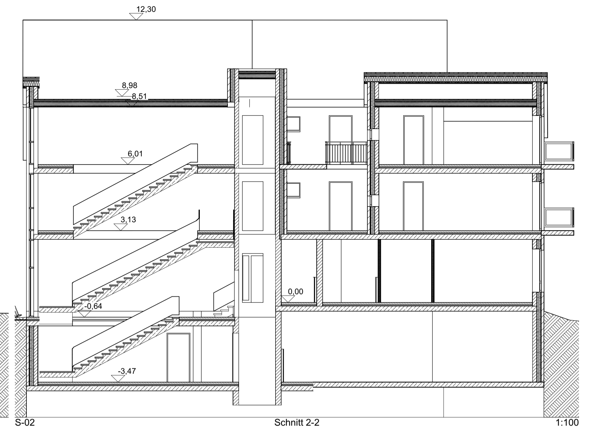
S-02 Schnitt 2-2 1:100
