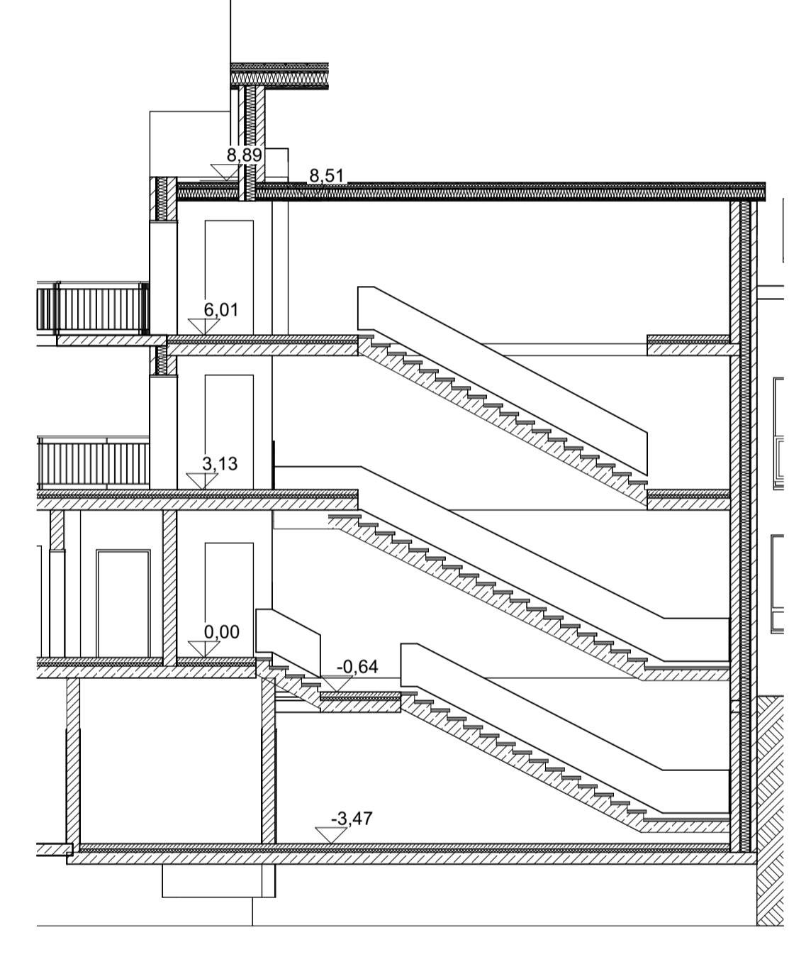
S-03 Schnitt 3-3 1:100
