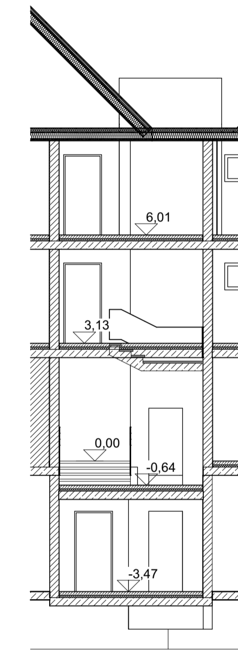
S-05 Schnitt 5-5 1:100
