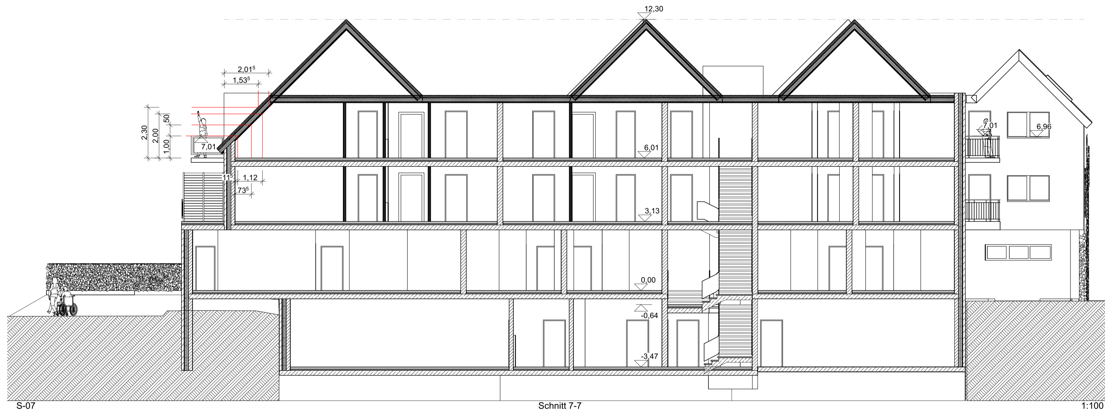
S-07 Schnitt 7-7 1:100
