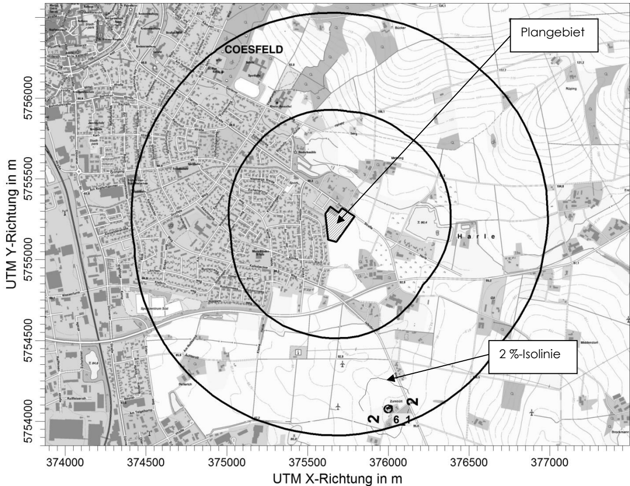
Abbildung 4: Zusatzbelastung IZ Nr. 6, genehmigter Bestand, Isolinien in % der Jahresstunden
