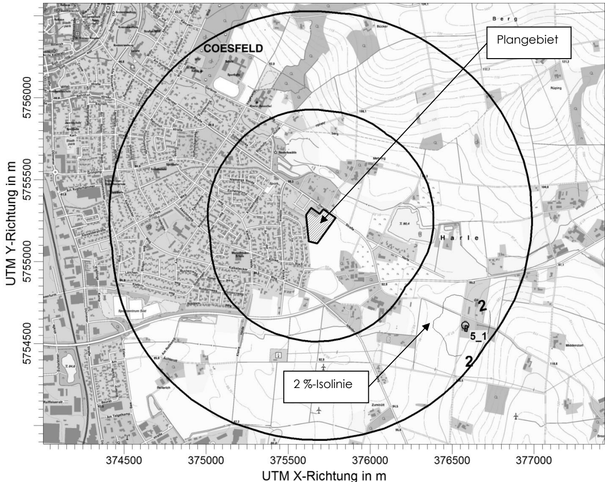
Abbildung 3: Zusatzbelastung IZ Nr. 5, genehmigter Bestand, Isolinien in % der Jahresstunden
