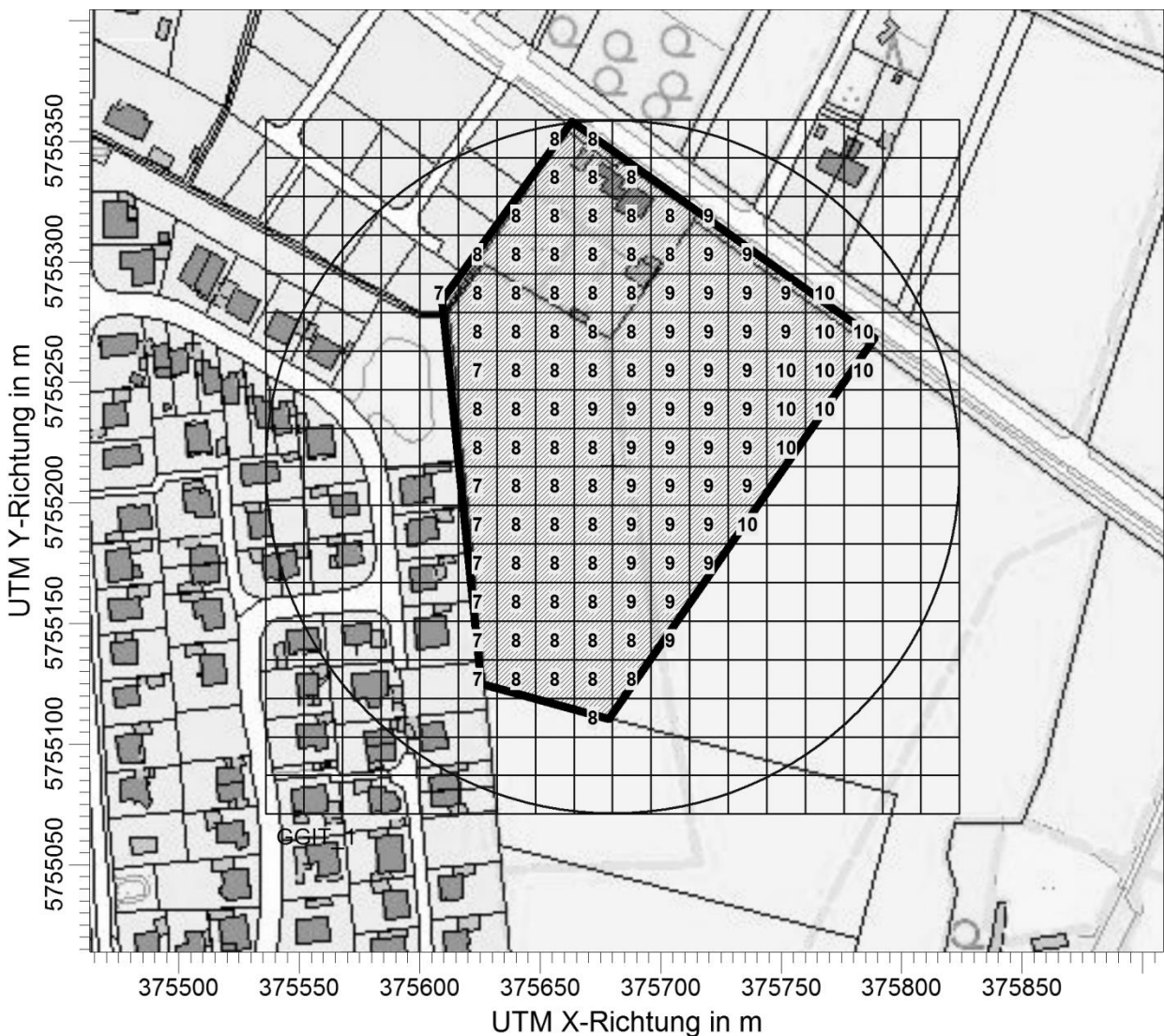
Abbildung 6: Gesamtbelastung IG b im genehmigten Bestand in % der Jahresstunden, Kantenlänge 16 m
