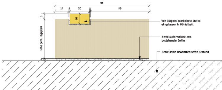
Berkelstein in Sohle M 1:10
