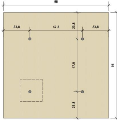
Untere Ansicht Berkelstein M 1:10
