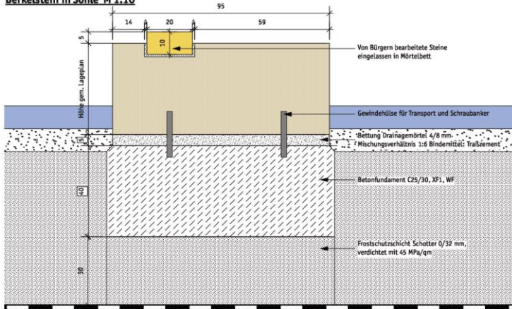
Berkelstein in Sohle M 1:10
