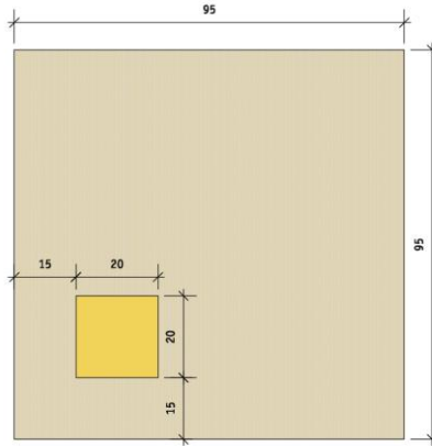
Berkelstein in Sohle Bestand M 1:10
