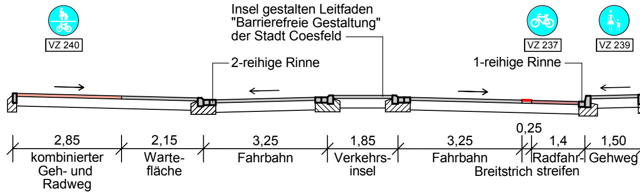
Schnitt c-c Planung
