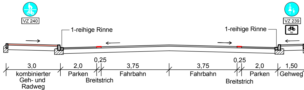
Schnitt c-c Bestand
