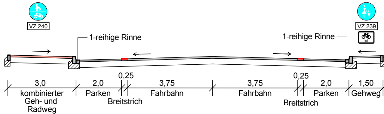
Schnitt a-a Bestand
