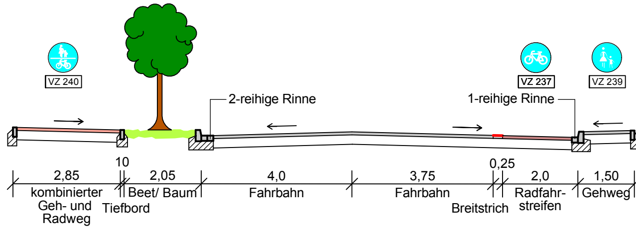
Schnitt a-a Planung
