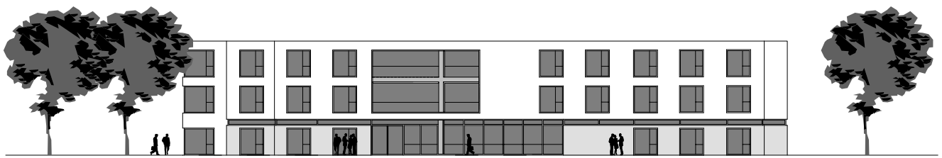
Ansicht von Süden, Altenpflegeheim M.1:200
