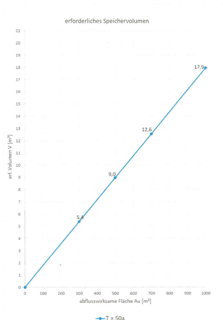
Abbildung: Speichervolumen in Anhängigkeit der abflusswirksamen Fläche
