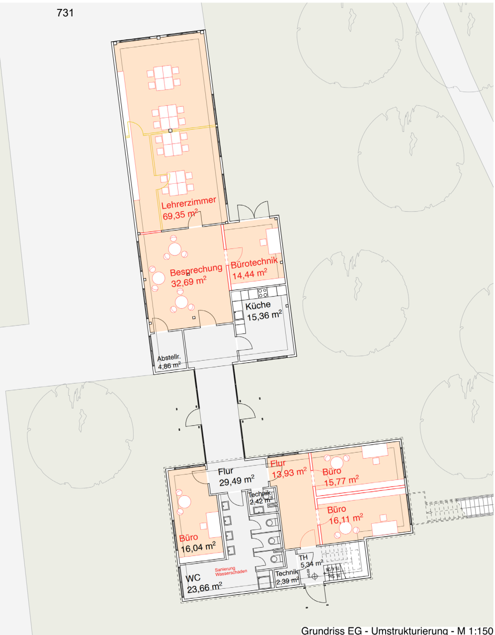
Grundriss EG - Umstrukturierung - M 1:150
