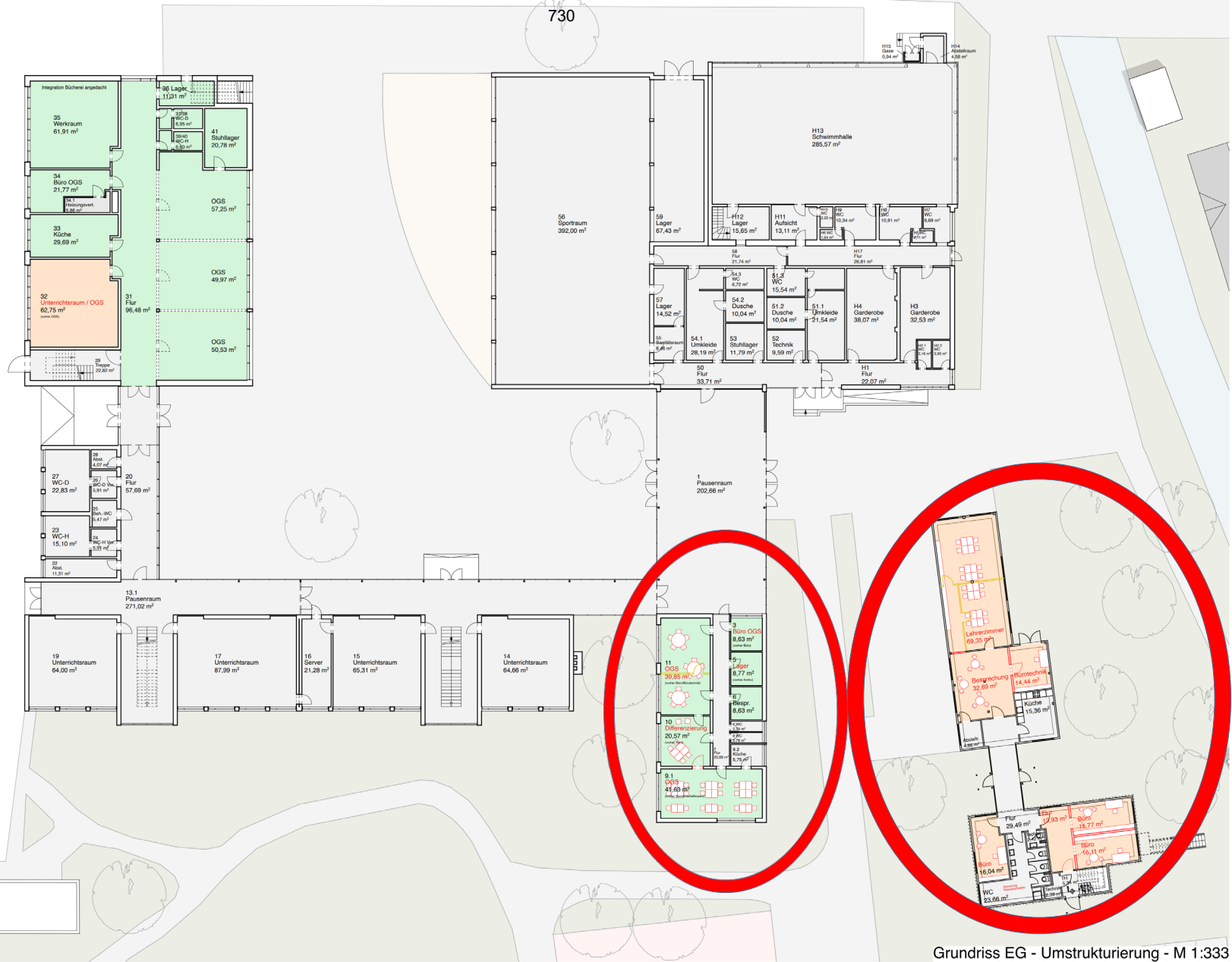
Grundriss EG - Umstrukturierung - M 1:333
