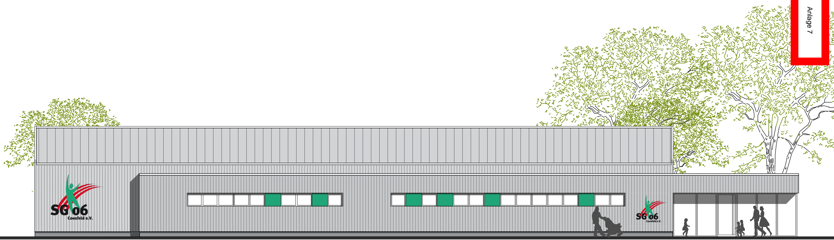
Ansicht Nord-Westen
