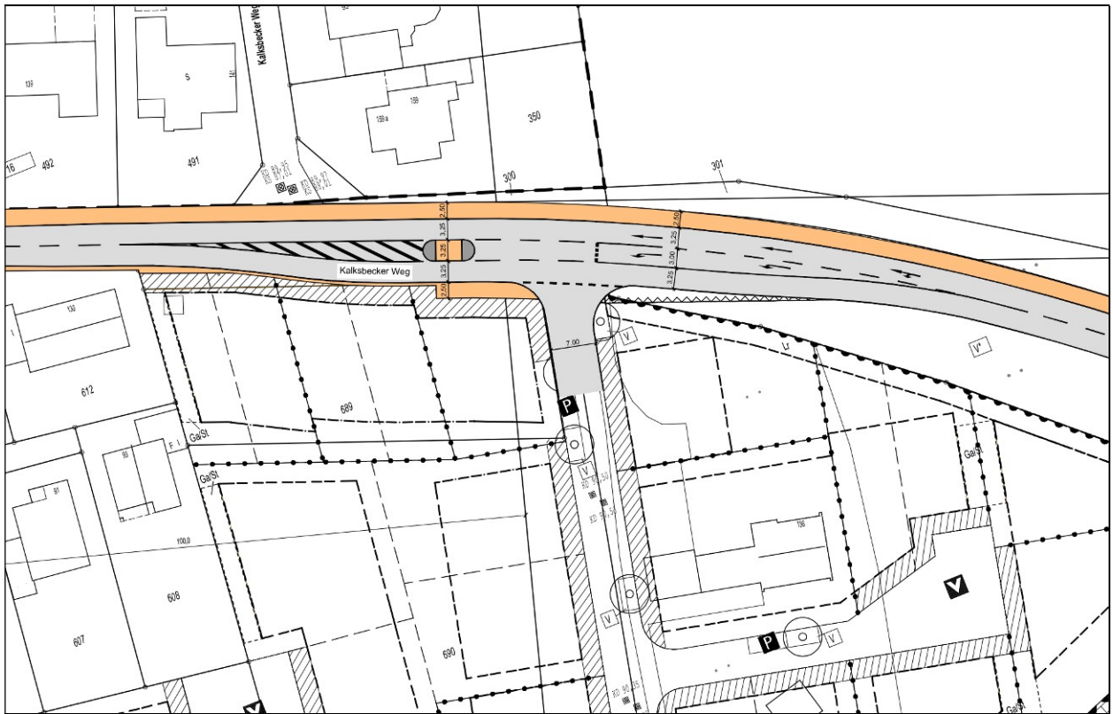
Abbildung 13: Verkehrstechnische Skizze – Anbindung Wohngebiet
